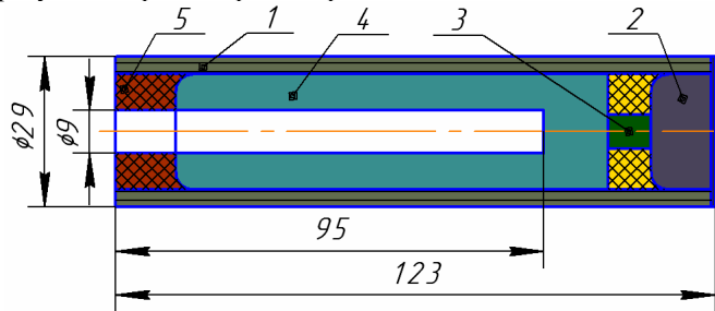
Рис 1 - схема двигателя РД1-50-5
